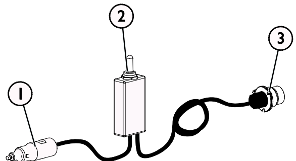
Kabelbundel A34731
